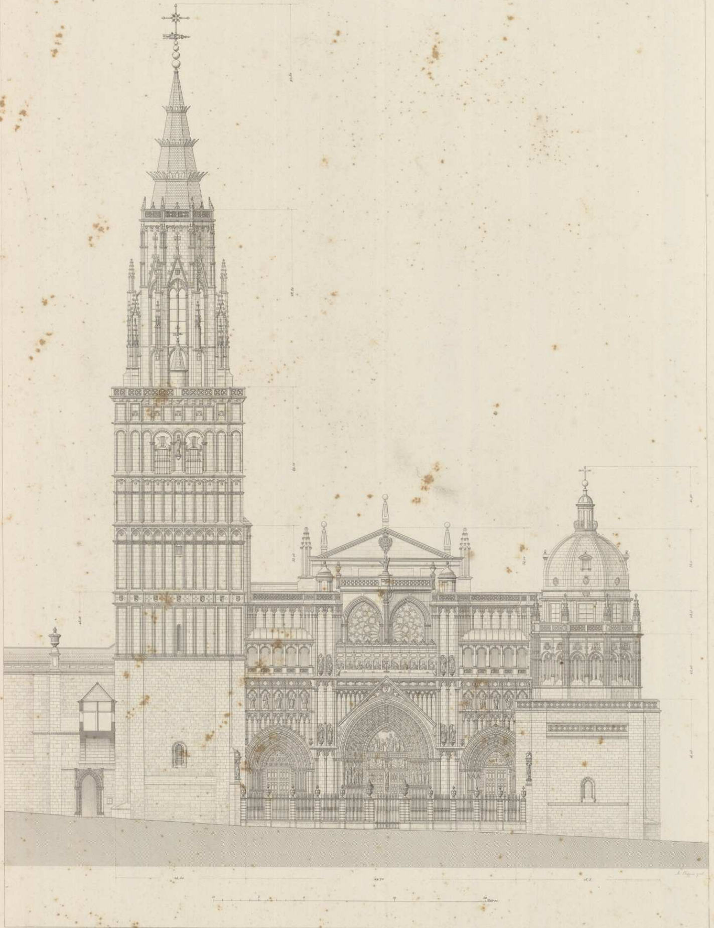
IMAFRONTA DE LA CATEDRAL, (TOLEDO).
