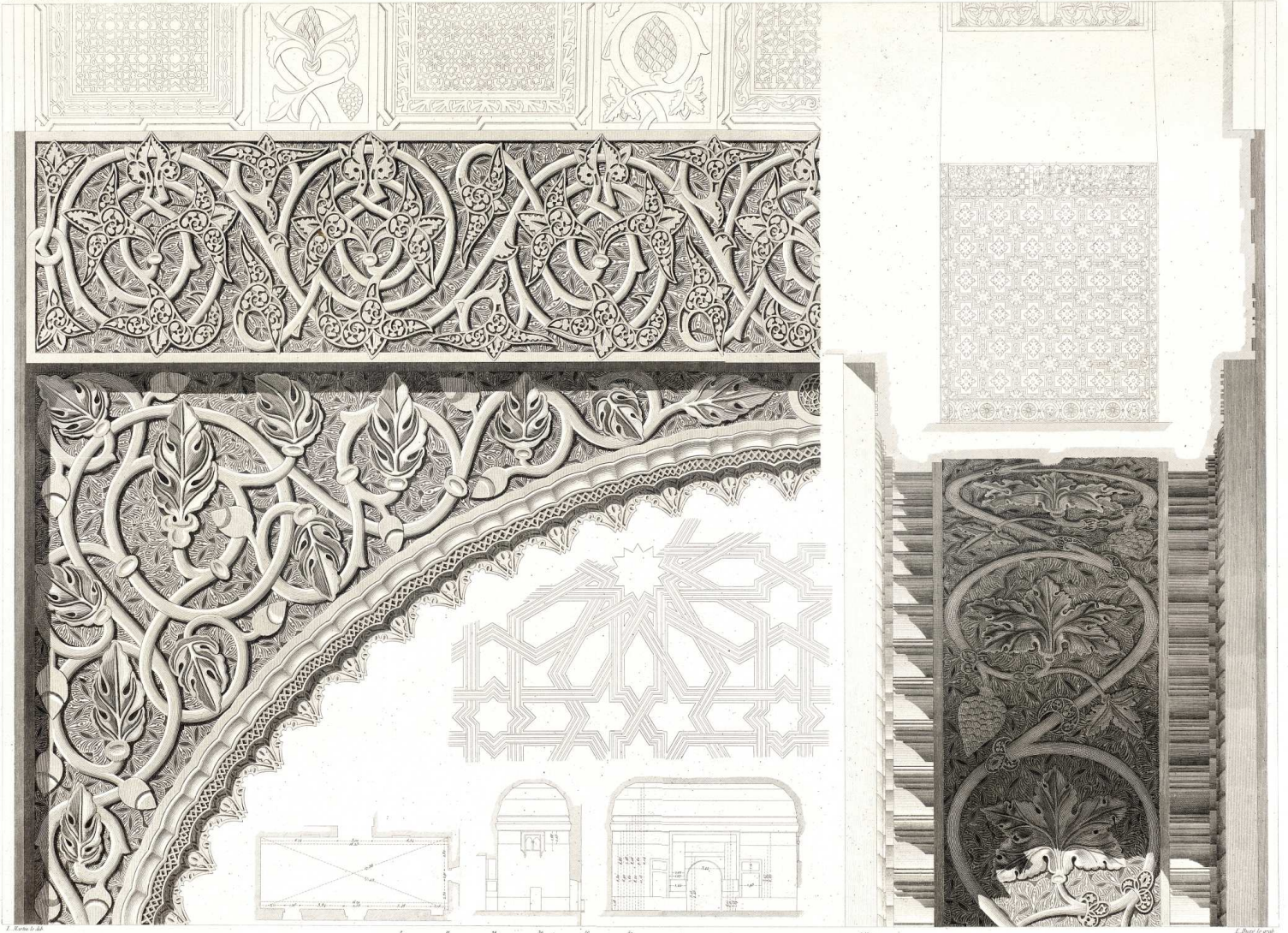
DETALLES DEL SALON DE LA CASA LLAMADA DE MESA. (TOLEDO.)
