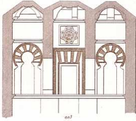
Seccion por la linea C D de la proyeccion horizontal.
