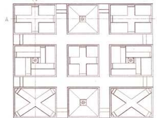
Proyeccion horizontal de las bóvedas del centro.
