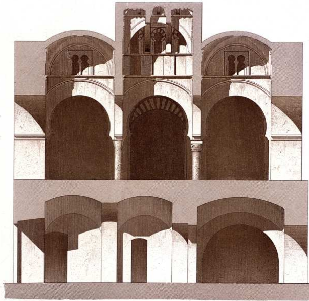
Seccion por la linea C D de la proyeccion horizontal.
