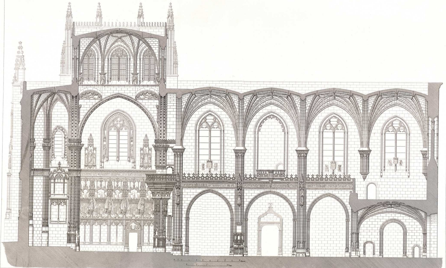
SECCION LONGITUDINAL DE LA IGLESIA DE SAN JUAN DE LOS REYES. (TOLEDO.)
