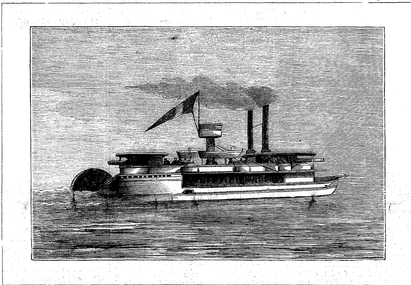
MARINA FRANCESA.—CAÑONERA RIVIERE, CONSTRUIDA PARA LAS OPERACIONES DEL TON-KIN.
