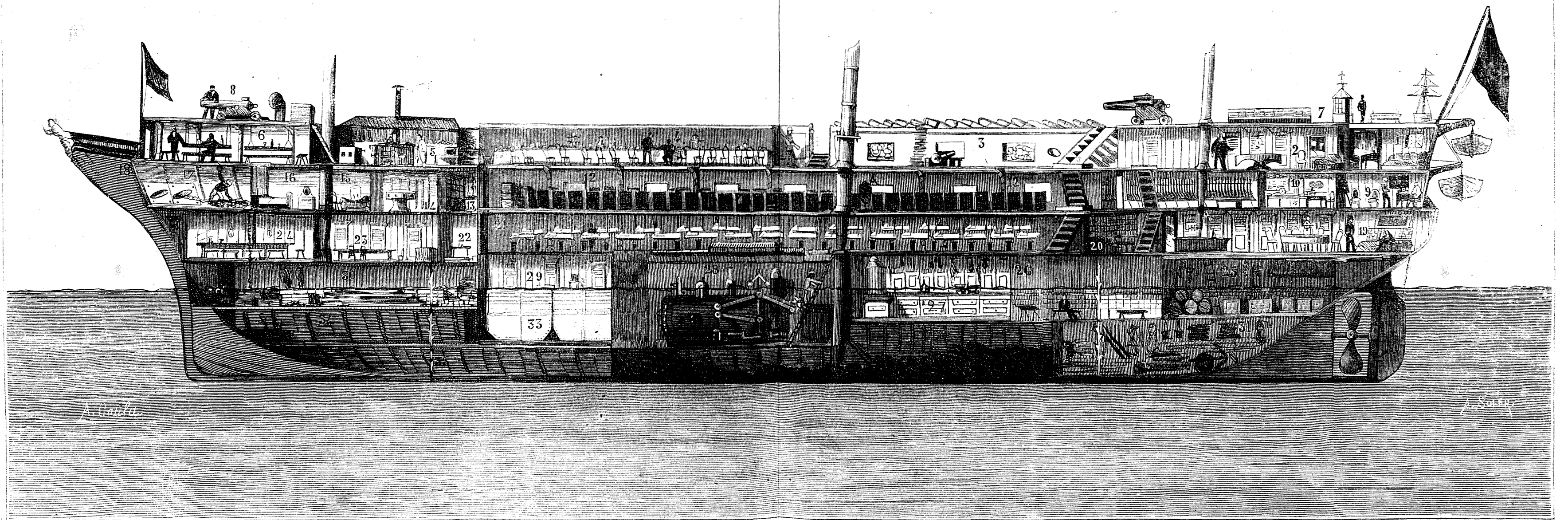
MARINA DE GUERRA.—FRAGATA ASTÚRIAS EN EL FONDEADERO DE LA GRAÑA, ESCUELA DE ASPIRANTES Á GUARDIAS MARINAS DE LA ARMADA.—1 Despacho del Comandante.—2 Cámara de los Jefes.—3 La cubierta y portalon.—4 Comedor de los alumnos.—5 Cocina.—6 Comedor de la marinería.—7 Observatorio y toldillo de popa.—8 Castillo de proa y colisa.—9 Aula de matemáticas.—10 Idem de física y química.—11 Sala de armas.—12 Sala de estudios.—13 Botica.—14 Un sobrestante.—15 Sala de baño.—16 Enfermería.—17 Los escobenes y cadena del ancla.—18 Jardines de proa.—19 Cámara de oficiales.—20 Biblioteca.—21 Dormitorio.—22 Sastrería.—23 Cámara de la maestranza.—24 Comedor de la Maestranza.—25 Nañol de la Santa Bárbara.—26 Calabozos.—27 La despensa.—28 Máquina.—29 Nañoles del Contramaestre y maquinista.—30 y 31 Almacén general.—32 Carbonera.—33 Algebres.—34 La barra.—35 La sentina.—A. Pizarra de Jorge Juan.
