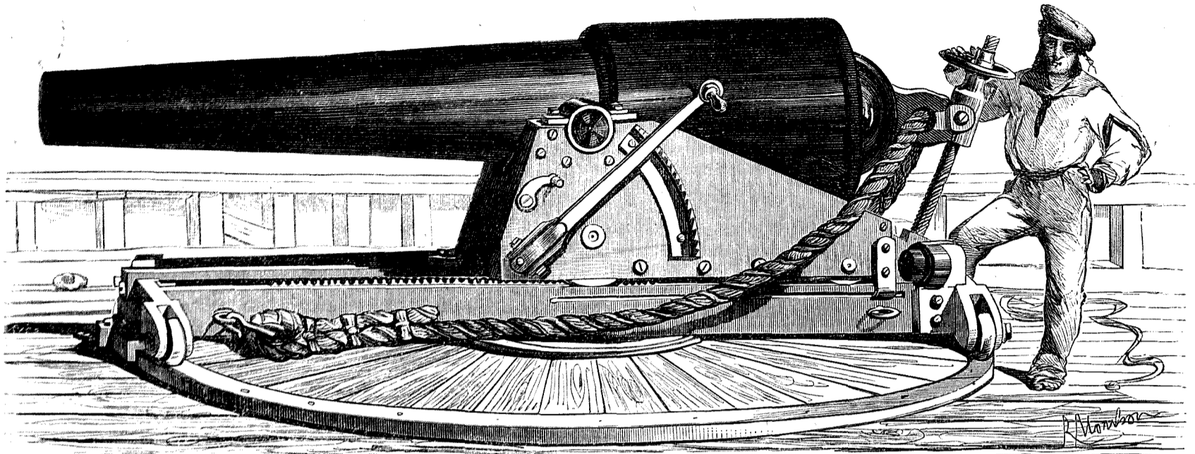
MODELO DEL CAÑON CONSTRUIDO POR M. ERICSSON PARA LAS CAÑONERAS ESPAÑOLAS.
