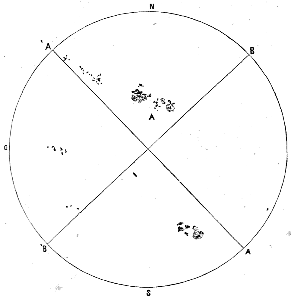
MANCHAS DEL SOL ESTUDIADAS EN EL OBSERVATORIO ASTRONÓMICO DE MADRID.
