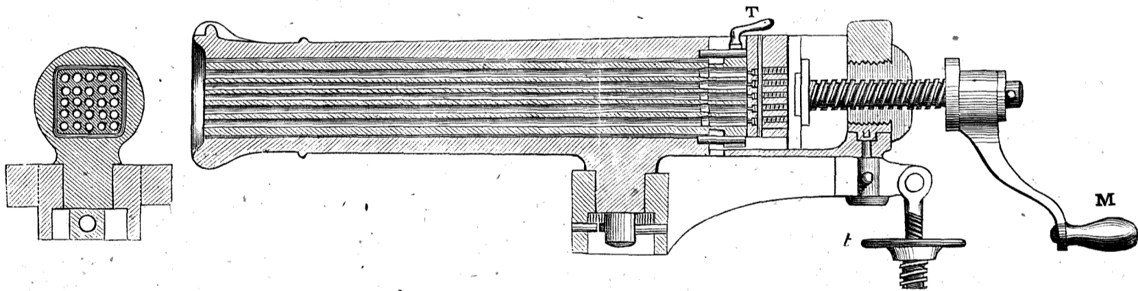
AMETRALLADORA FRANCESA DEL SIGLO XIX
