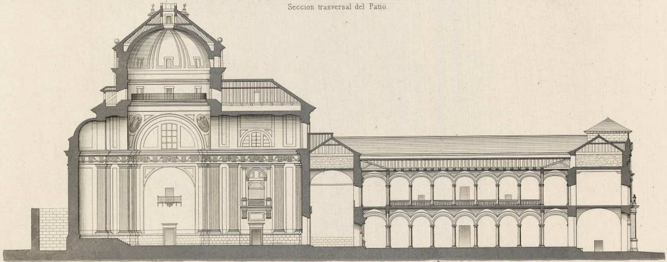
Seccion longitudinal
