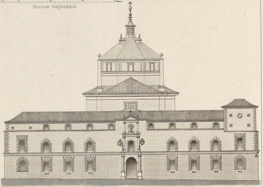
Alzado
