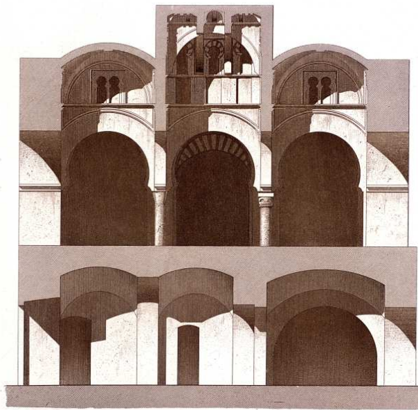
Seccion por la linea C D de la proyeccion horizontal.
